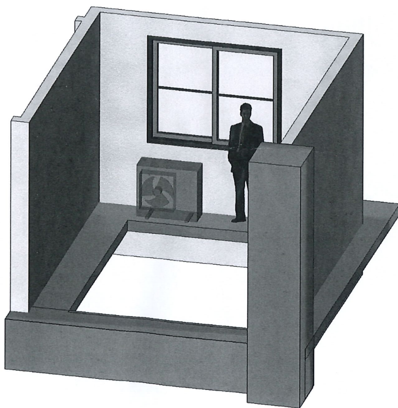
圖 3-4-1、天井安裝室外機錯誤範例-1
