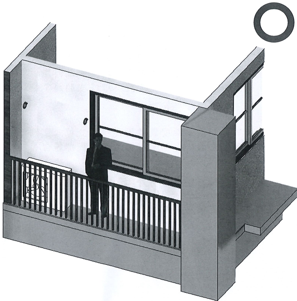
圖 2-2、露樑設置室外機範例
